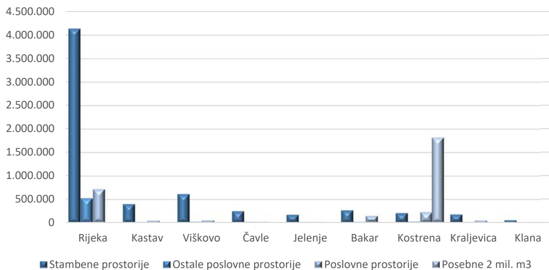
Grafikon 2: Količina vodne usluge javne vodoopskrbe po gradovima i općinama u m 3 za I-IX 2023.
