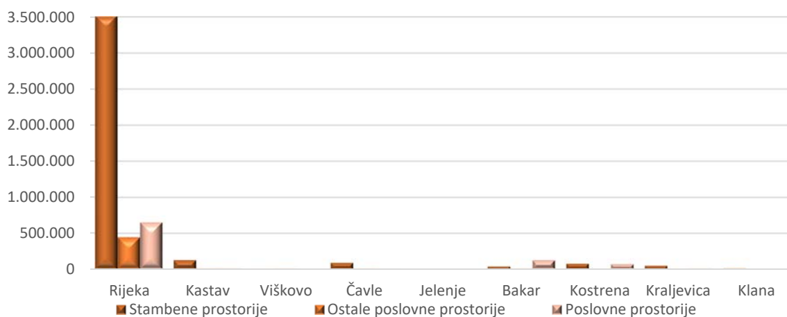
Grafikon 5: Količina vodne usluge javne odvodnje - skupljanje I otpadne vode po gradovima i općinama u m 3 za I-IX 2023.
